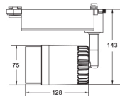
A-4 12W/15W
